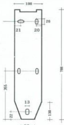
PENSILINE SPORGENZA 2000 / 1750
