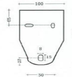
PENSILINE SPORGENZA 1000 / 750
