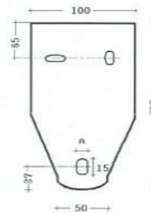
PENSILINE SPORGENZA 1500 / 1250
