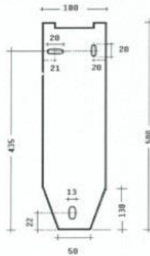
PENSILINE SPORGENZA 1100 / 1300 / 1500
